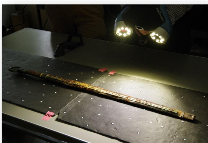
姉崎 山王山古墳出土 金銀装単龍環頭大刀の計測
